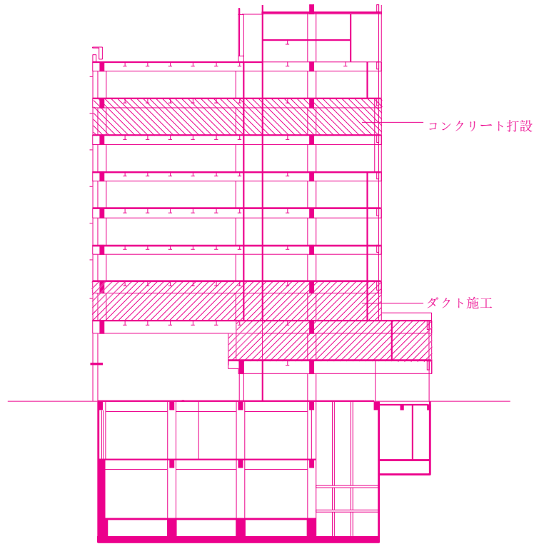
断面図
