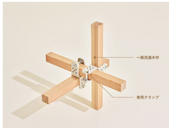
つな木のしくみ。一般流通木材と専用クランプを活用。
